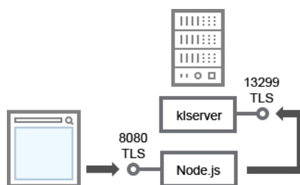
Сервер администрирования и Kaspersky Security Center 13 Web Console
