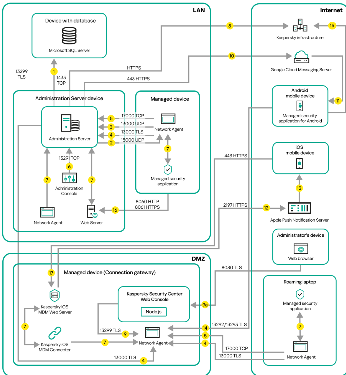
Управляемые мобильные устройства, подключенные к Серверу администрирования через шлюз соединения
