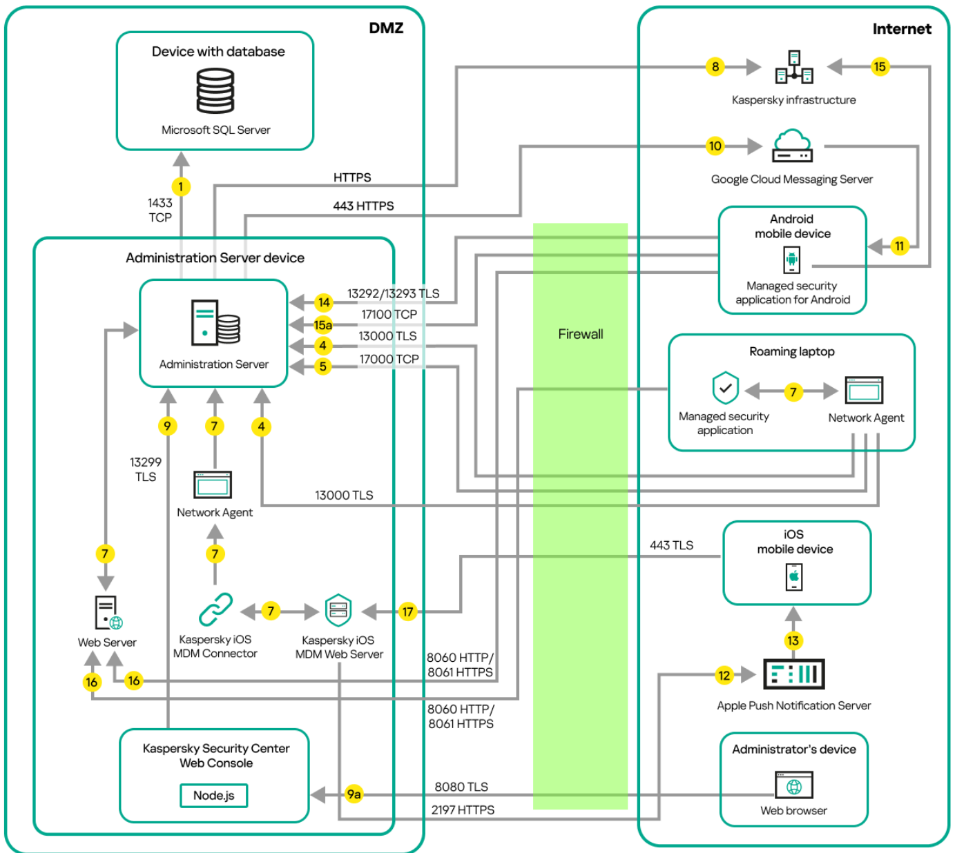
Сервер администрирования в локальной сети; управляемые устройства подключаются к Серверу администрирования с помощью корпоративного сетевого экрана
