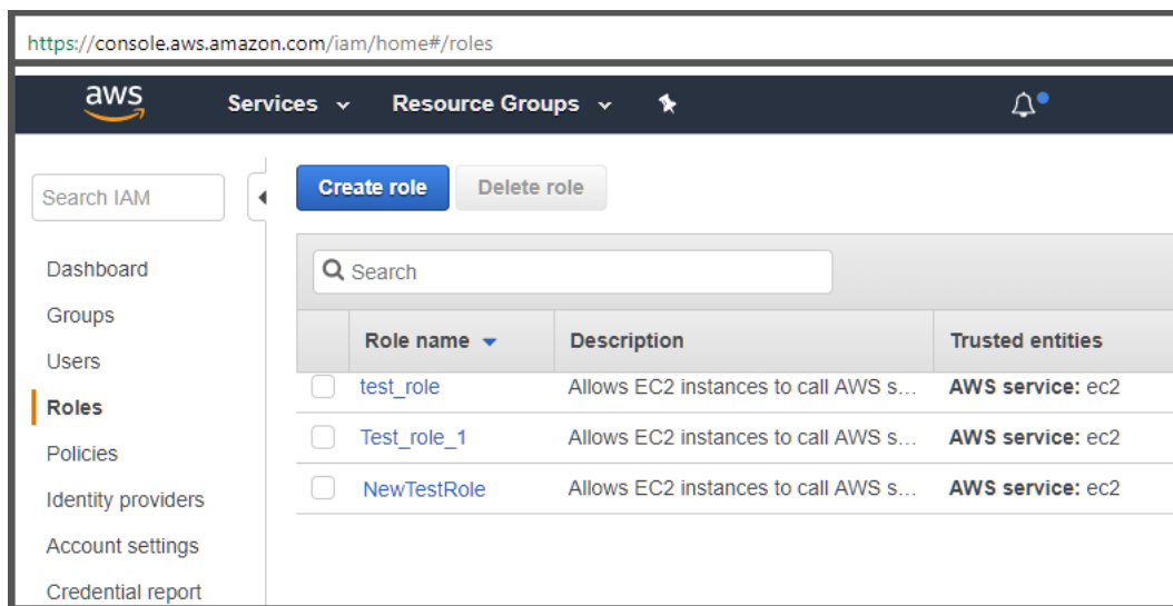
Создание IAM-роли в Консоли управления AWS
