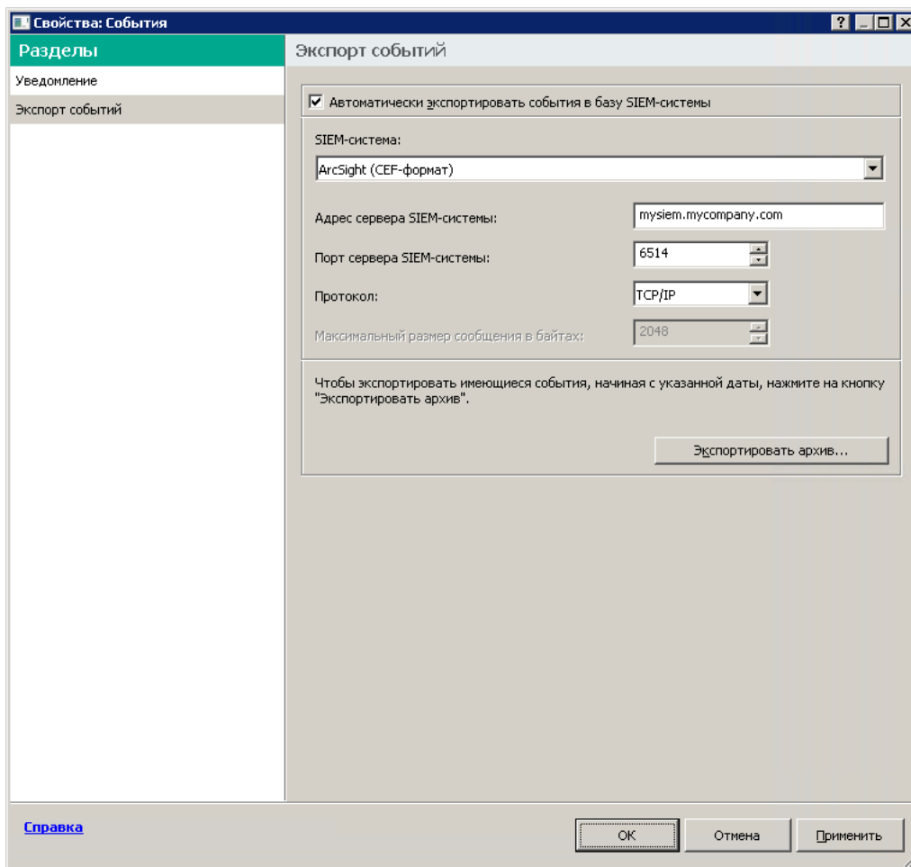
Раздел Экспорт событий окна свойств событий
