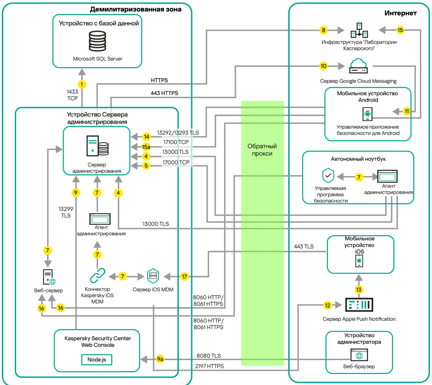
Сервер администрирования в локальной сети; управляемые устройства подключаются к Серверу администрирования с помощью обратного прокси-сервера
