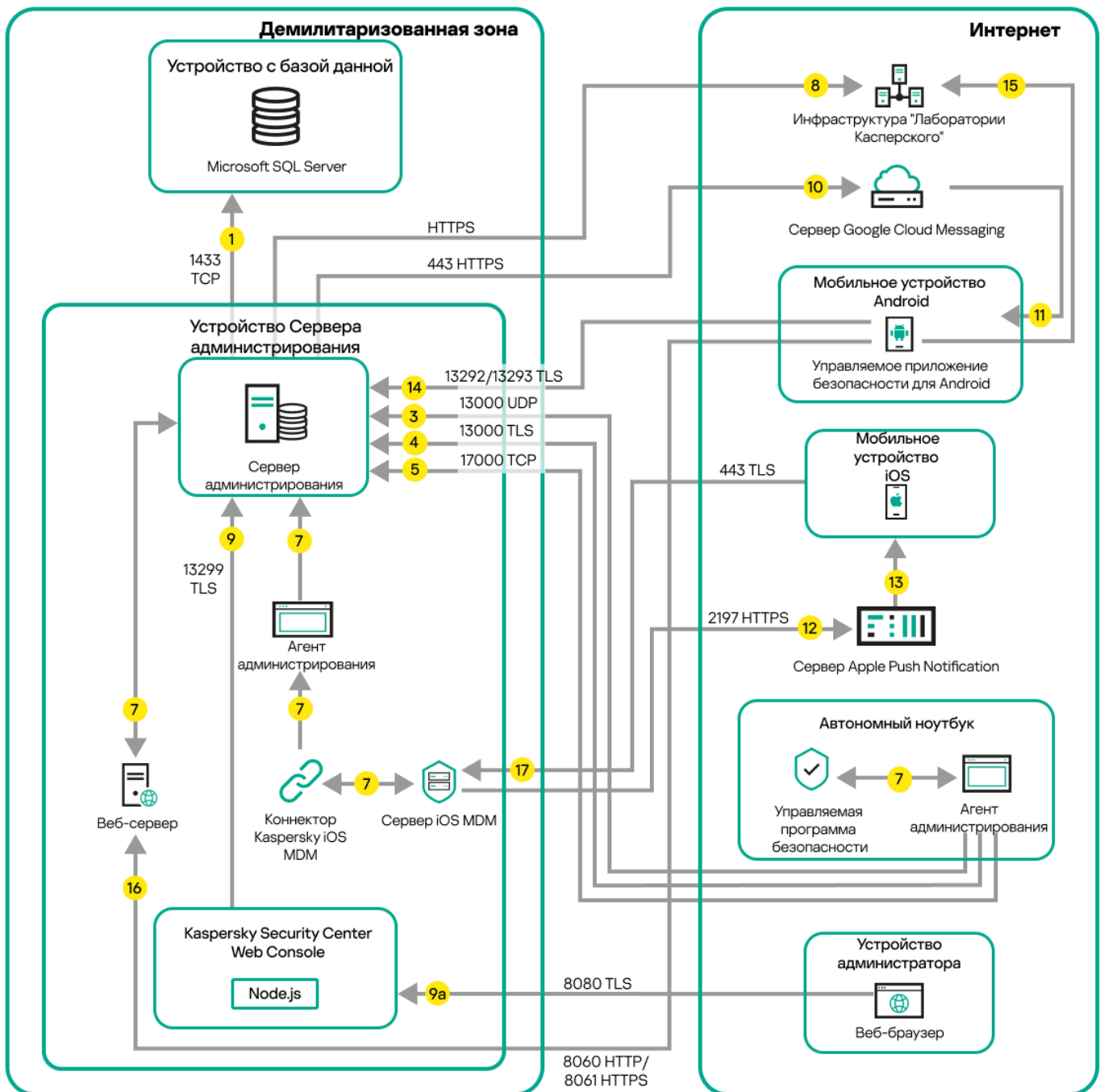
Сервер администрирования в демилитаризованной зоне, управляемые мобильные устройства в интернете
