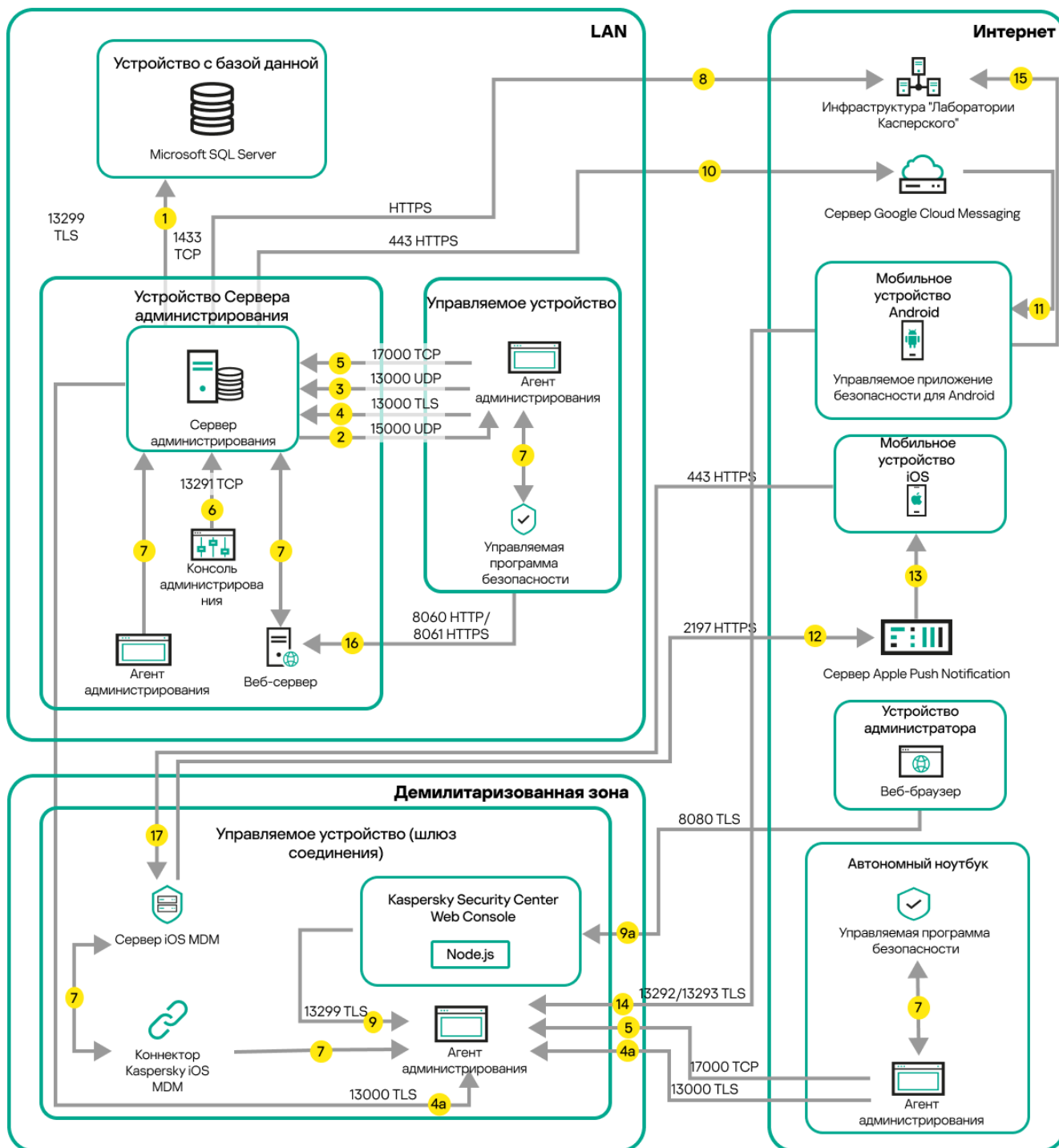
Управляемые мобильные устройства, подключенные к Серверу администрирования через шлюз соединений
