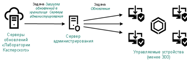
Обновление с использованием задачи Загрузка обновлений в хранилище Сервера администрирования и без точек распространения
