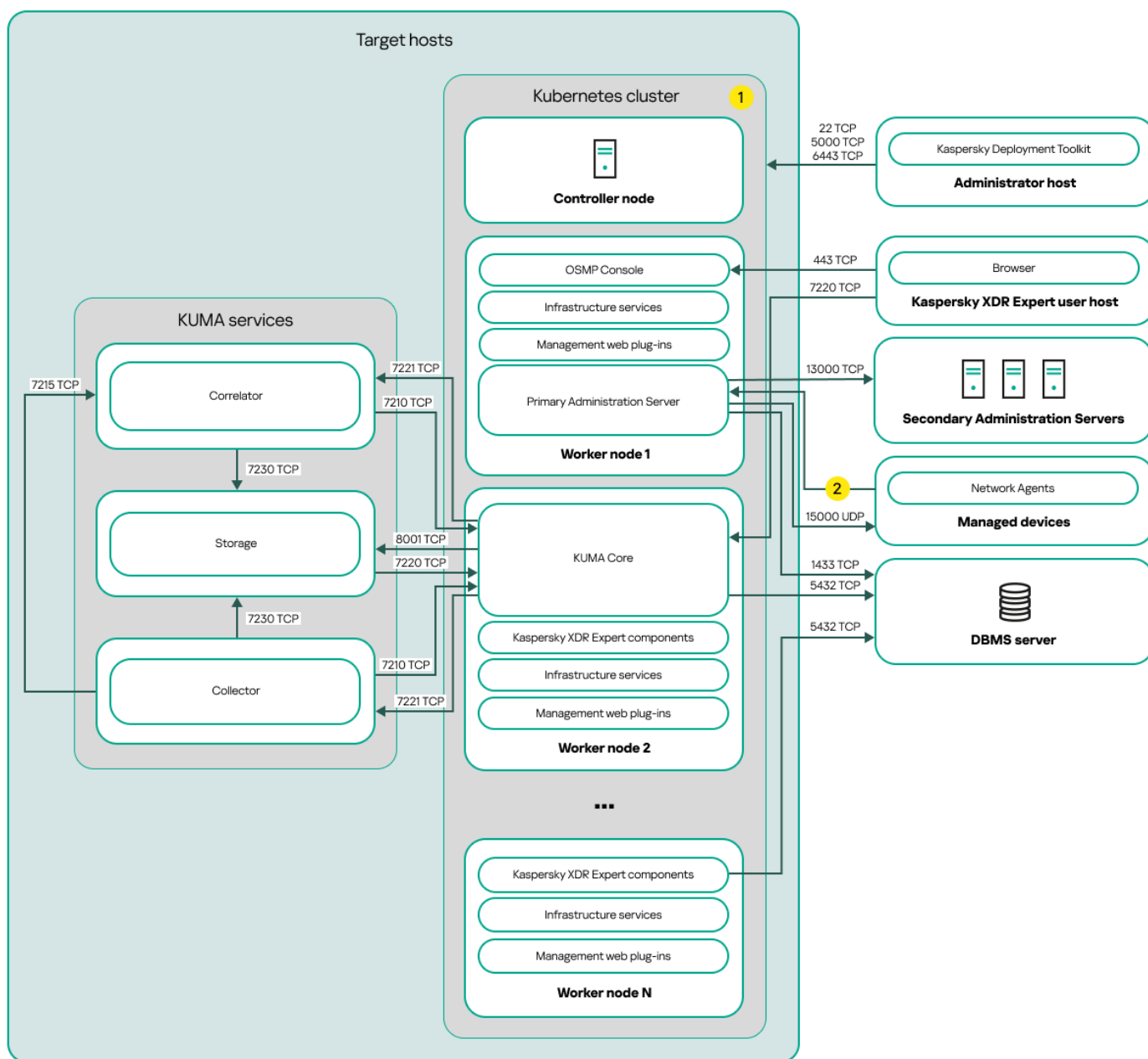
Схема распределенного развертывания Open Single Management Platform
